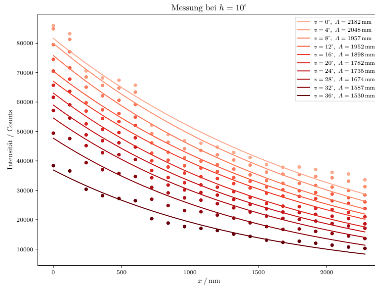
Abbildung 8: Die gemessenen Intensitäten für einen festen horizontalen Winkel h = 10^\circ und verschiedenen vertikalen Winkeln v von 0^\circ bis 36^\circ und verschiedenen x -Werten von 0 mm bis 2400 mm.
